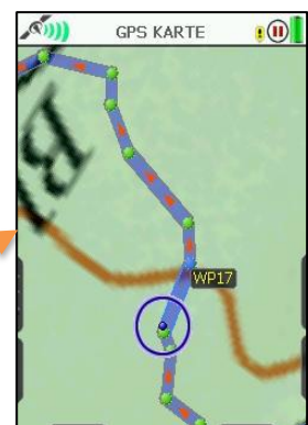
GPS Karte
