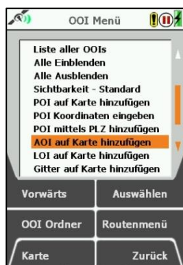
Menüpunkt wählen
