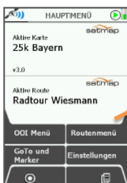
Hauptseite "Hauptmenü"
