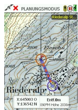
Anzeige GoTo-Route
